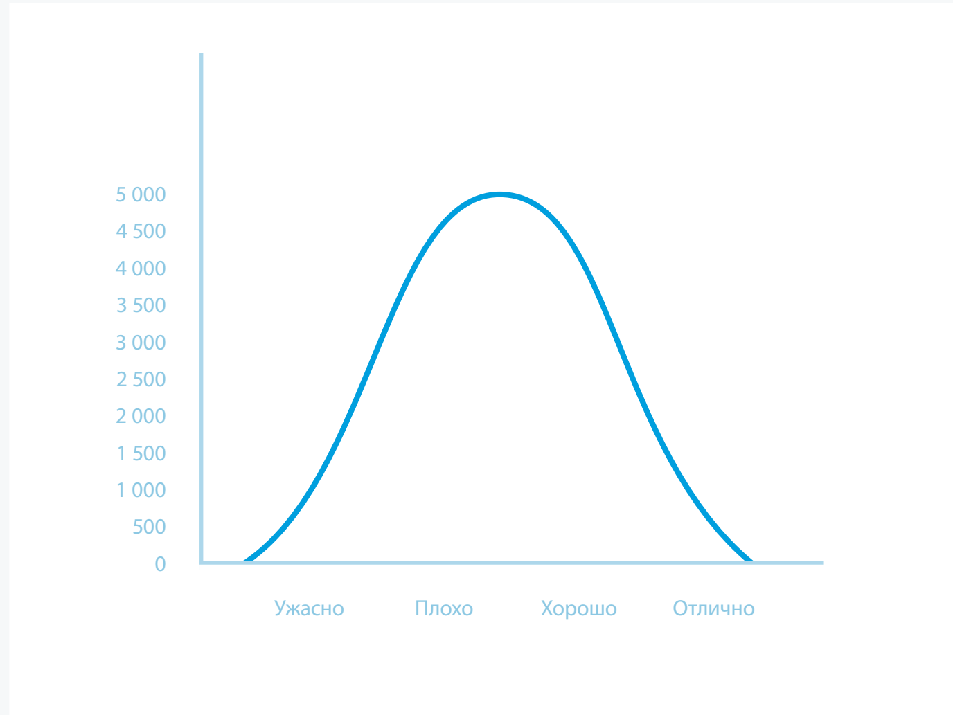
Нормальное распределение. Зависимость количества голосов от оценки по категории опроса (например оценка качества услуг общественного транспорта)
